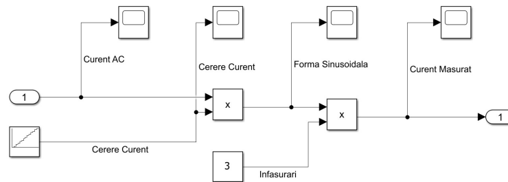
Figura 14. Schemă bloc a curentului de intrare în sistem
